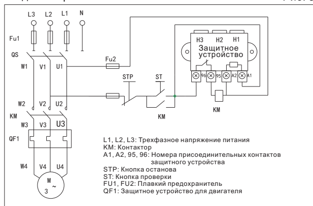
7.2 На рис. 3 показана схема соединений цепи управления для напряжения 380 и 400 В. Рис. 3
