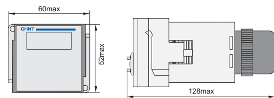
Размер отверстия
