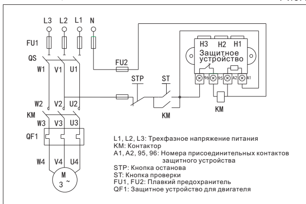
7.1 На рис. 2 показана схема соединений цепи управления для напряжения 220 и 230 В. Рис. 2
