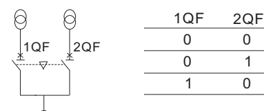
Схема коммутации. Возможные комм. состояния.
